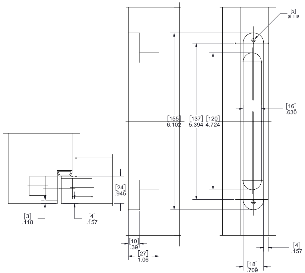
Milling Door
